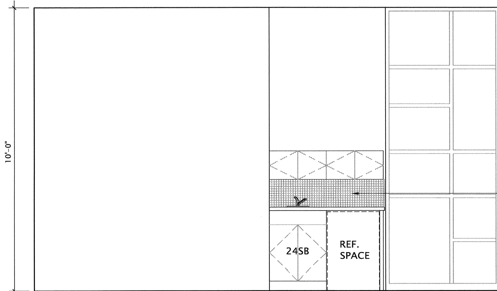
A1 LIVING ROOM SCALE: 1/2" = 1'-0"
